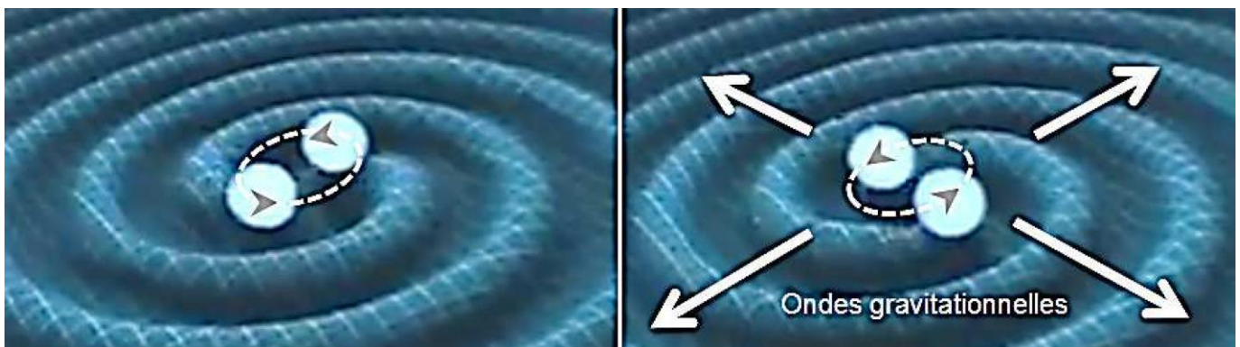
Illustration de l'émission d'ondes gravitationnelles lors de la rotation d'un couple de trous noirs de même masse.
