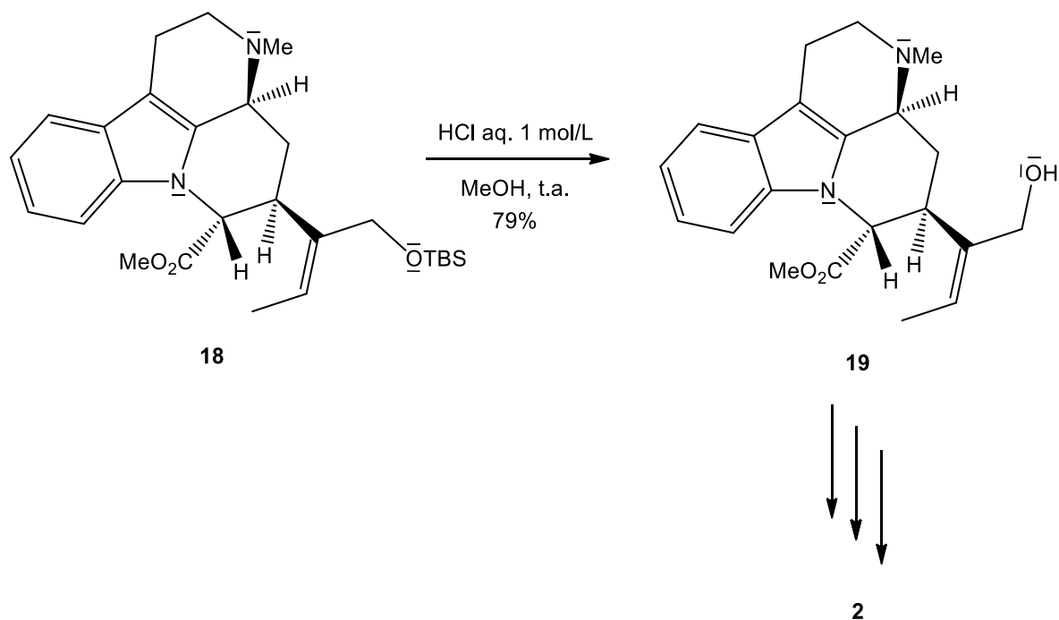
Figure 9 – Schéma réactionnel de la synthèse de 19 à partir de 18.
