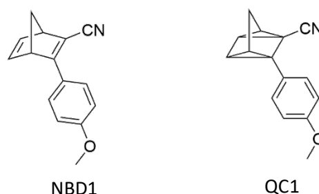
Figure 12 – Structure des composés NBD1 et QC1.
