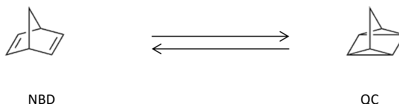
Figure 11 – Structure des composés NBD et QC et réaction d'isomérisation.
