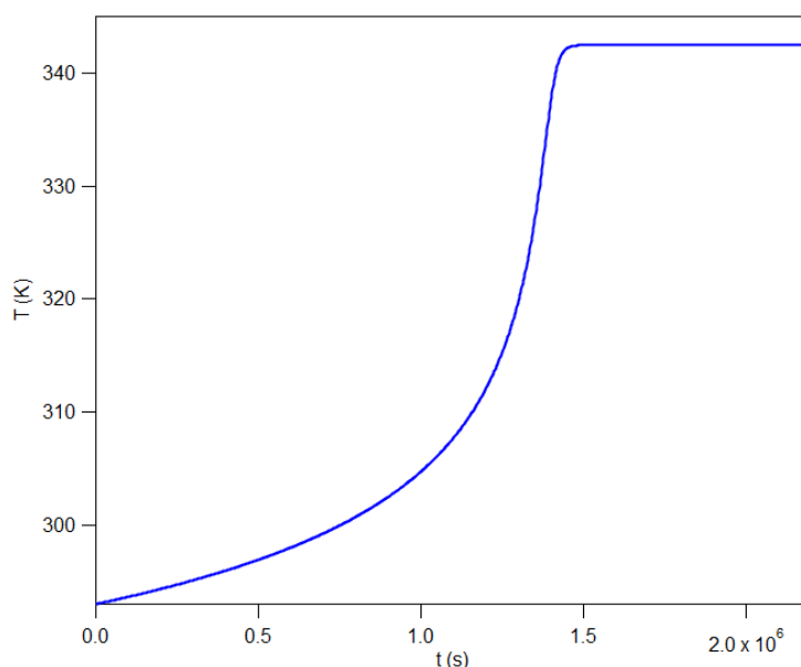
Figure 16 – Simulation de la temp  rature    l'int  rieur du calorim  tre au cours du temps, pour une temp  rature initiale de 20   C.
