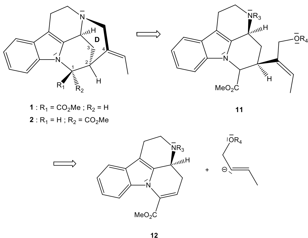
Figure 5 – Schéma rétrosynthétique de la synthèse des alcaloïdes 1 ( R_1 = \text{CO}_2\text{Me} et R_2 = \text{H} ) et 2 ( R_1 = \text{H} et R_2 = \text{CO}_2\text{Me} ) à partir du précurseur 12 .
