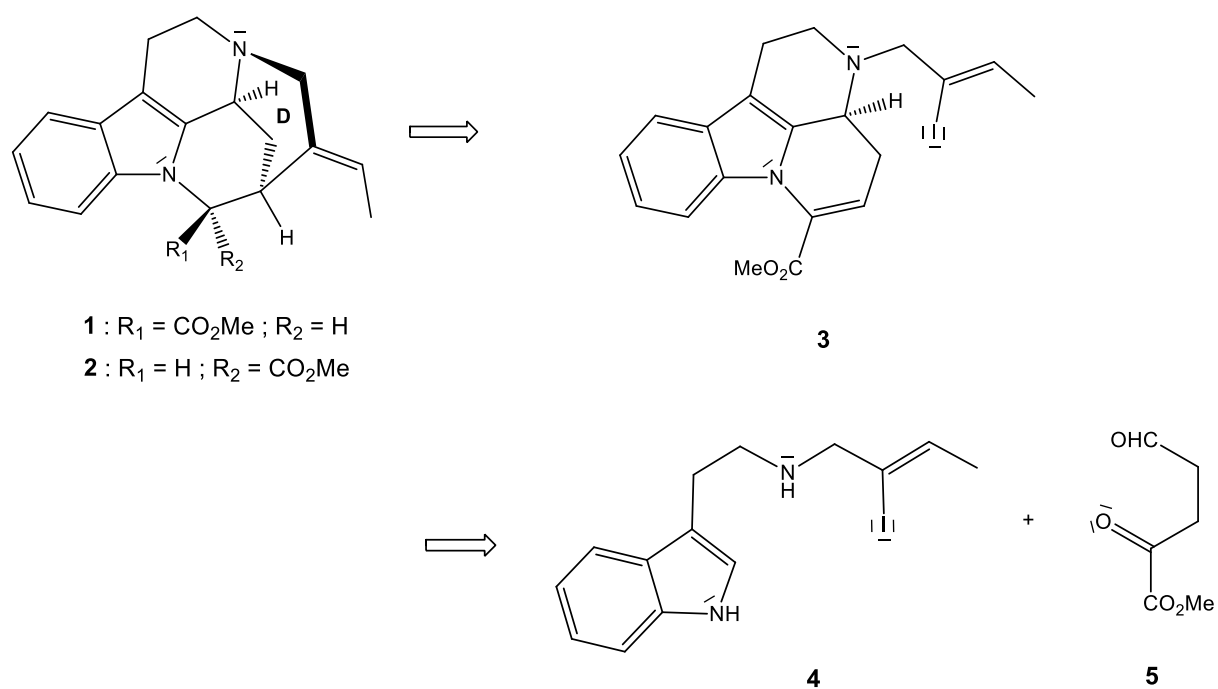
Figure 1 – Schéma rétrosynthétique de la synthèse des alcaloïdes 1 ( R_1 = \text{CO}_2\text{Me} et R_2 = \text{H} ) et 2 ( R_1 = \text{H} et R_2 = \text{CO}_2\text{Me} ) à partir des précurseurs 4 et 5 .
