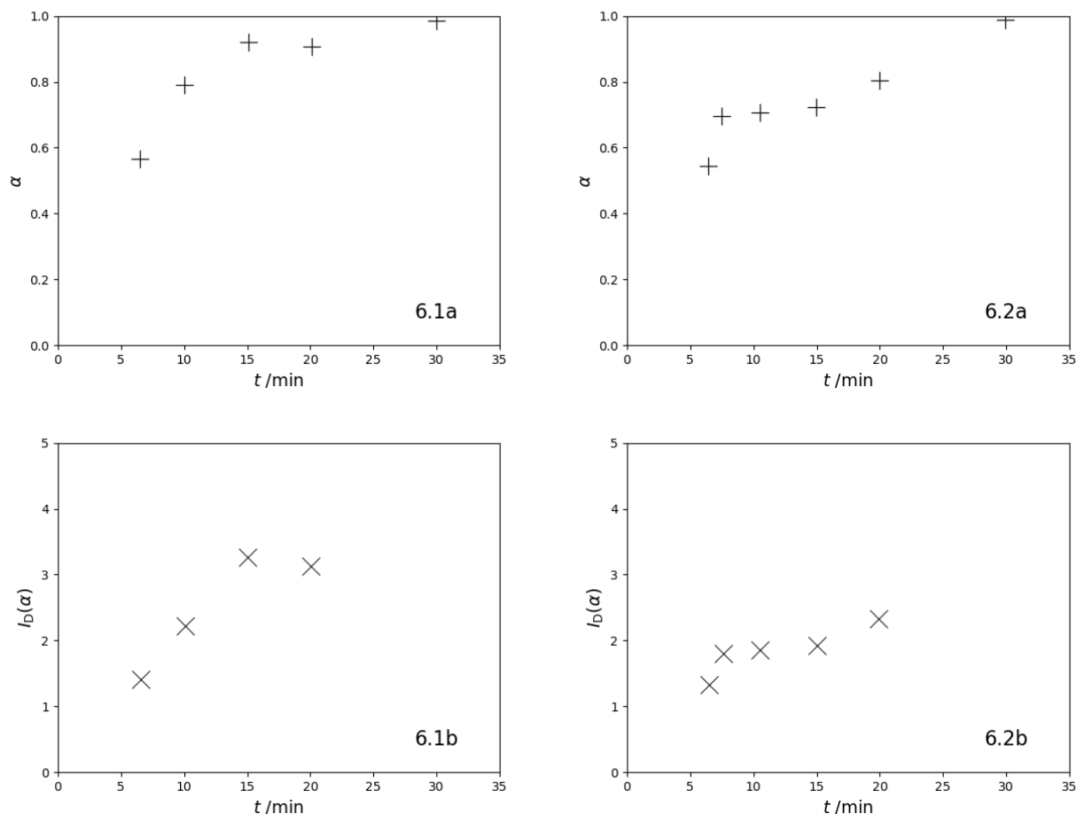
Figure 6 : évolution du degré de cristallisation \alpha (+) et du paramètre chronomètre I_D(\alpha) (x) en fonction du temps pour deux concentrations de travail initiales différentes
