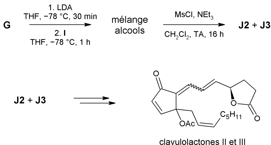
Figure 15 : troisième partie de la synthèse étudiée
