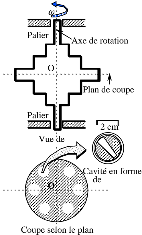
Fig. 1 : schéma de principe du rotor d'une ultracentrifugeuse
