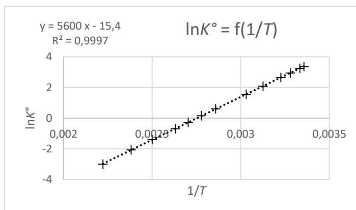
Figure 1-c : Évolution de \ln(K^\circ) en fonction de l'inverse de la température
