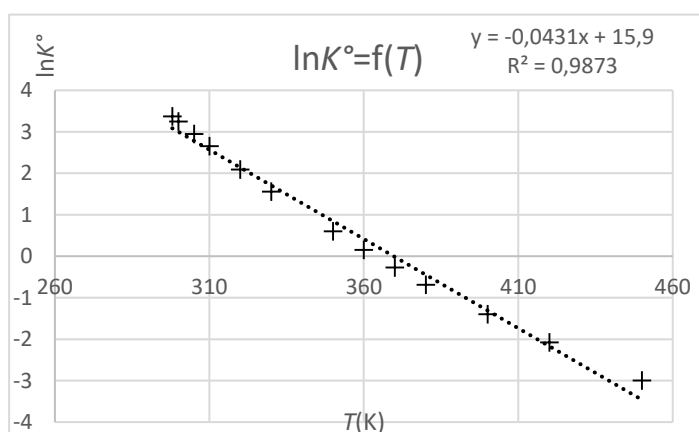
Figure 1-b : Évolution de \ln(K^\circ) en fonction de la température.
