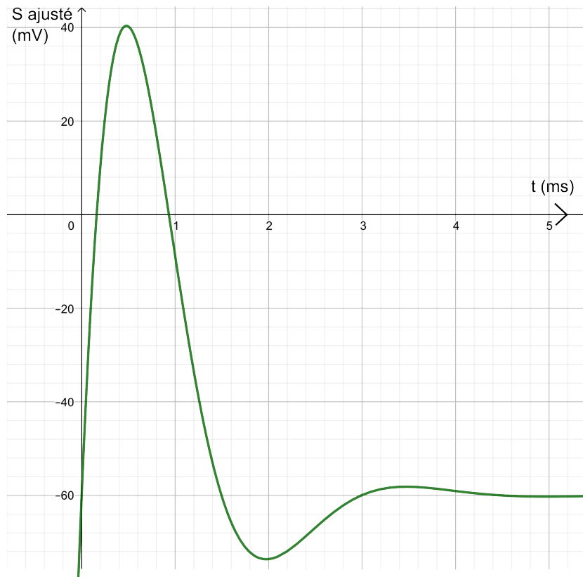
FIGURE 8 – Signal S ajusté en choisissant les paramètres A , \tau et \omega de façon à se rapprocher au mieux de l'allure du potentiel d'action. Les valeurs retenues sont A = 225 mV, \tau = 0.75 s, et \omega = 2.1 rad·s -1 .
