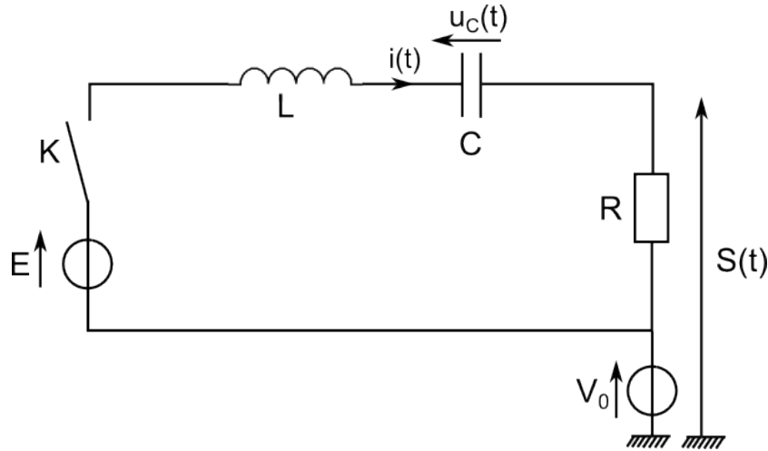
FIGURE 7 – Circuit RLC soumis à un échelon de tension. On cherche les valeurs de V_0 , E , R , L et C telles que le signal S(t) du circuit corresponde le plus possible au signal S(t) du neurone.
