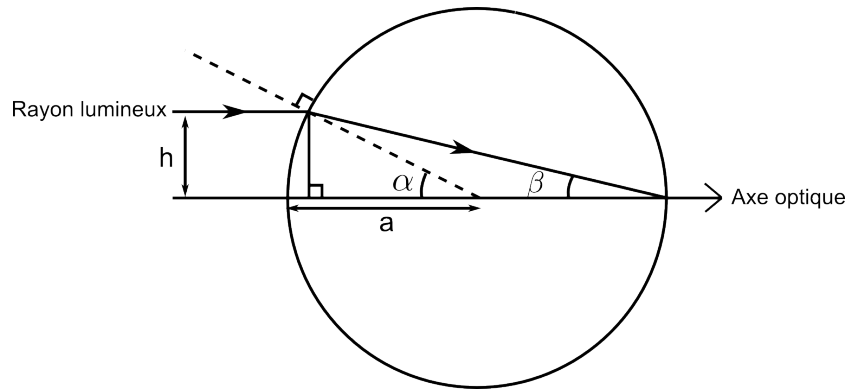
FIGURE 3 – Rayons venant de l’infini traversant l’oeil modélisé par une sphère d’indice n .
