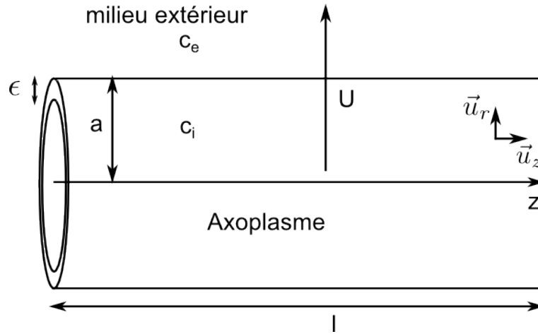
FIGURE 5 – Modèle d'axone cylindrique.
