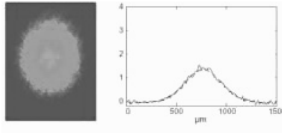
FIG. 1 – Profil de densité optique d'un nuage de rubidium après une expansion libre de 20 ms. À droite : coupe du profil de densité.
