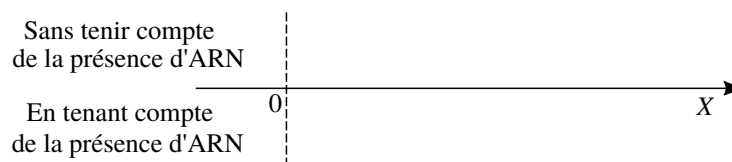
FIGURE 2 – Domaines de formation des virus, selon la valeur du paramètre X = \kappa/\kappa^* (graphe à reproduire et compléter).
