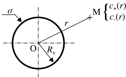
FIGURE 1 – Coque virale dans une solution ionique.
