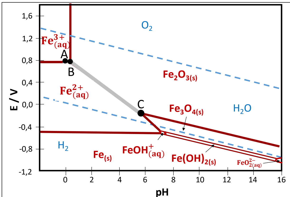
Figure 4 - Diagramme E-pH du fer pour C_{\text{tracé}} = 1 \text{ mol.L}^{-1} . À la frontière entre deux espèces dissoutes (aq) : les concentrations des deux espèces sont égales et leur somme est égale à C_{\text{tracé}} . À la frontière entre une espèce dissoute et un solide, la concentration de l'espèce dissoute vaut C_{\text{tracé}} ( T = 25^\circ\text{C} ).
