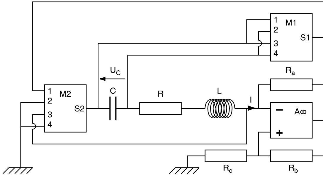
FIGURE 4 – M1 et M2 sont deux multipliers idéaux. A_{\infty} est un amplificateur opérationnel idéal, fonctionnant dans le régime linéaire.
