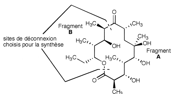
Erythronolide B
