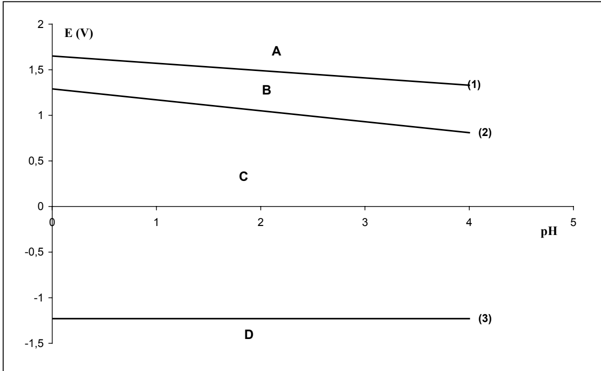
FIGURE 1 : Diagramme potentiel-pH simplifié du manganèse (concentration de tracé 10^{-2} \text{ mol.L}^{-1} ) :
