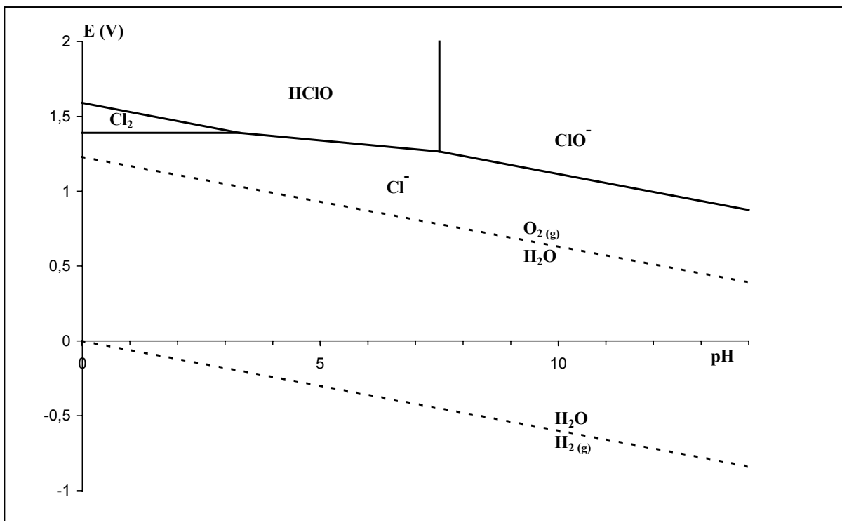
FIGURE 2 : Diagramme potentiel-pH du chlore (concentration de tracé 1 \text{ mol.L}^{-1} ) et diagramme potentiel-pH de l'eau :
