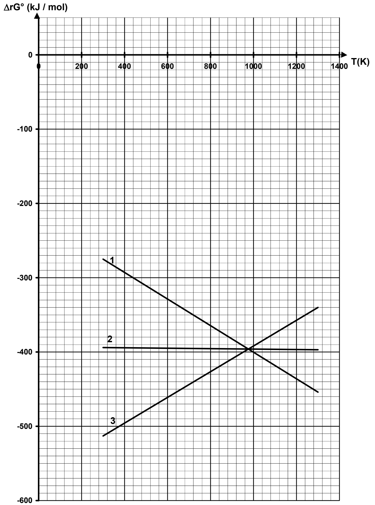
FIGURE I : Diagramme d'Ellingham des oxydes (rapporté à 1 mole de O 2 )
