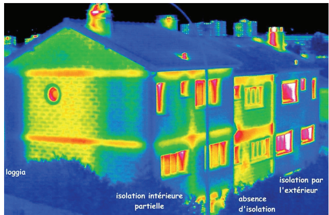
FIGURE 1 – Thermographie infrarouge.
