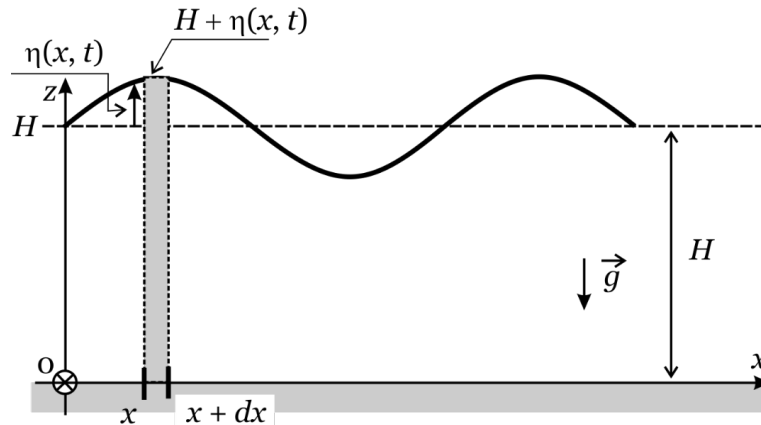
FIGURE 22 - Schéma d'ensemble.
