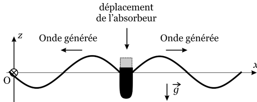
FIGURE 14 – Ondes créées par le mouvement vertical de l'absorbeur.
