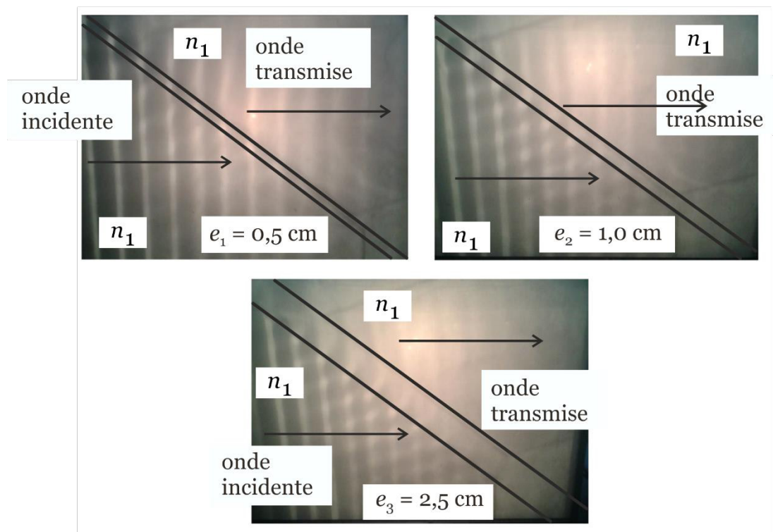
FIGURE 13 - Propagation de l'onde incidente dans la cuve en fonction de la largeur e de la zone d'indice n_2 .
