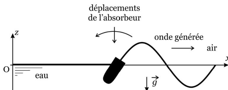
FIGURE 16 – Onde créée par la superposition du mouvement vertical et de la rotation de l'absorbeur.
