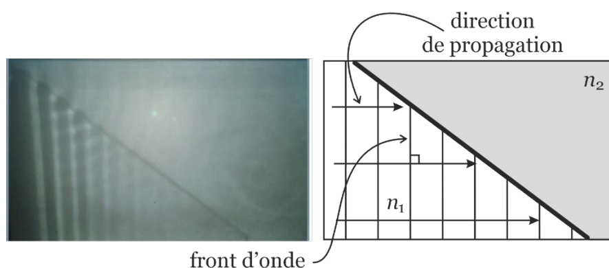
FIGURE 11 – Ondes observées dans le cas d'une incidence de 50^\circ .
