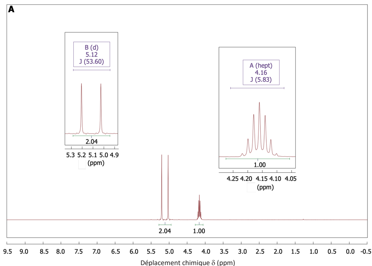
Fig. 1 – Spectre de RMN ^1\text{H} (300 MHz) du sévoflurane. Sur les agrandissements des massifs, les constantes de couplage J sont données en Hz.
