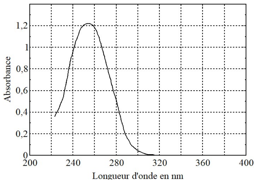
Figure 1 – Spectre d'absorption d'une solution d'ozone.
