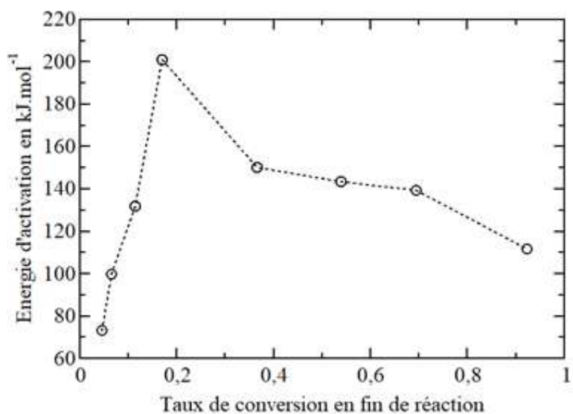
Figure 3 – Évolution de l'énergie d'activation en fonction du taux de conversion en fin de réaction (la courbe en pointillés a pour unique but de faciliter la visualisation de l'évolution)
