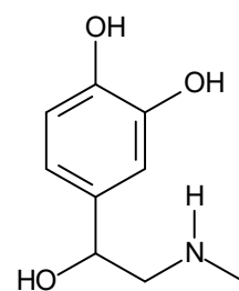
Figure 4 – Formule topologique de l'adrénaline
