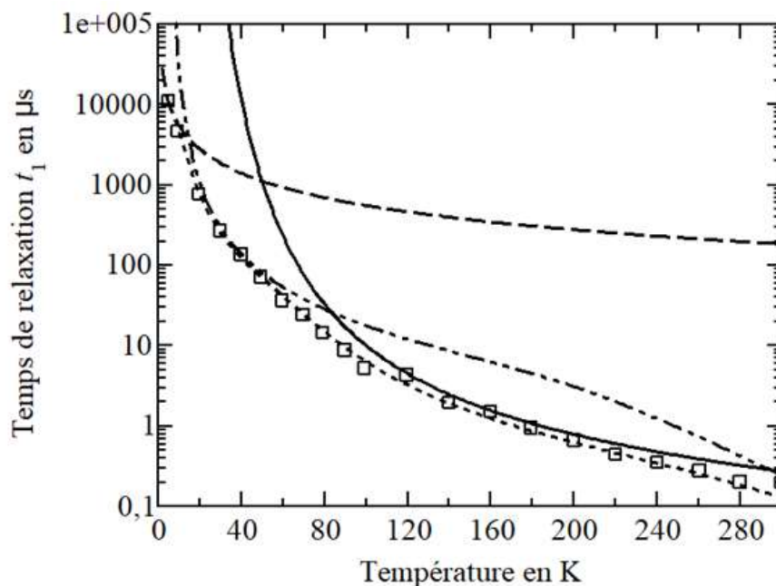
Figure 10 – Temps de relaxation t_1 en fonction de la température.
