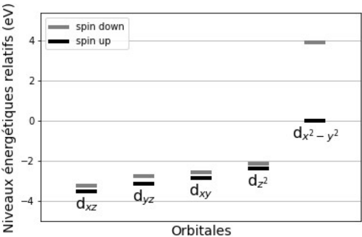
Figure 8 – Diagrammes des énergies relatives des orbitales d du cuivre dans le complexe 2. L’orbitale la plus énergétique de spin up est prise en référence d’énergie nulle.
