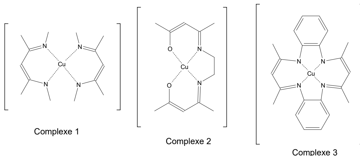
Figure 7 – Structures de trois complexes candidats qubit
