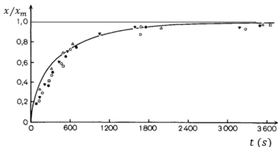
Figure 3 : Dépendance de l'épaisseur normalisée x' = x/x_m en fonction du temps pour des rapports constants des réactifs hexaméthylène diamine A et chlorure de sébacoyl C. C_c = 1,0 \text{ mol. L}^{-1} et (\square): C_A = 0,5 ; (\blacktriangledown): C_A = 0,3 ; (\bullet): C_A = 0,18 ; (\circ): C_A = 0,1 ; (\triangle): C_A = 0,05 \text{ mol. L}^{-1} . La ligne continue est obtenue à l'aide du modèle développé dans cette section.
