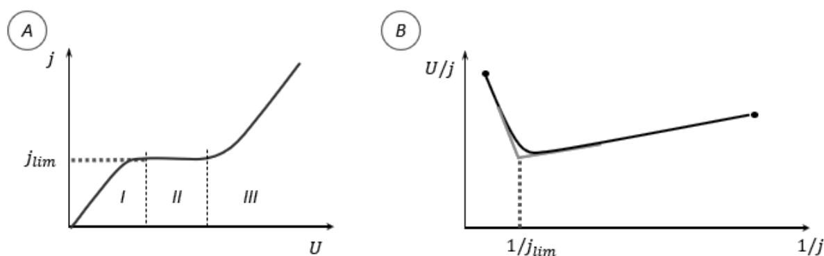
Figure 14 : A- Courbe densité de courant - tension pour une cellule électrolytique en écoulement dont les compartiments sont séparés par une membrane échangeuse d'ion. B- Représentation de Cowan-Brown U/j = f(1/j) pour la détermination expérimentale de j_{lim} .
