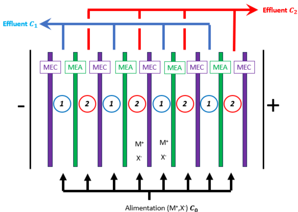
Figure 13 : Schéma d'une unité d'électrodialyse
