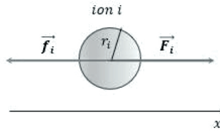
Figure 12 : Forces qui s'exercent sur un ion i dans un gradient de potentiel électrochimique à une dimension.
