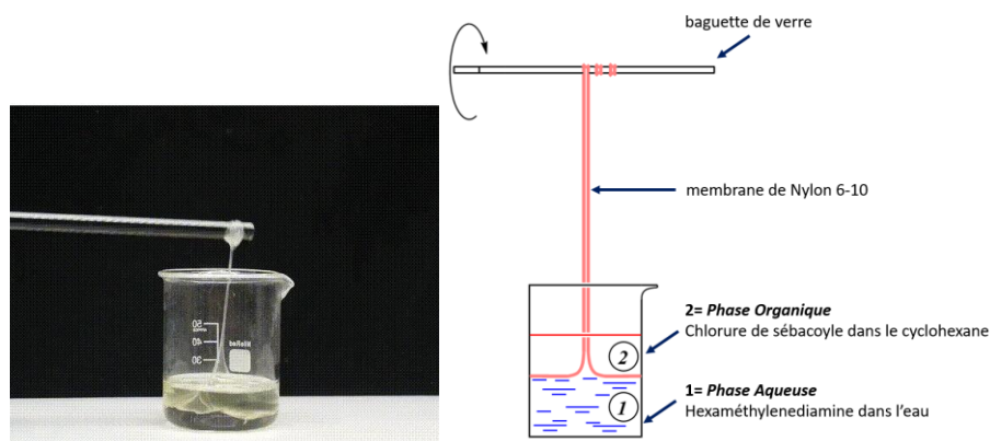
Figure 1 : Expérience de la corde de Nylon. La membrane qui se forme à l'interface entre les phases organique et aqueuse est continûment retirée et enroulée sur une baguette de verre.
