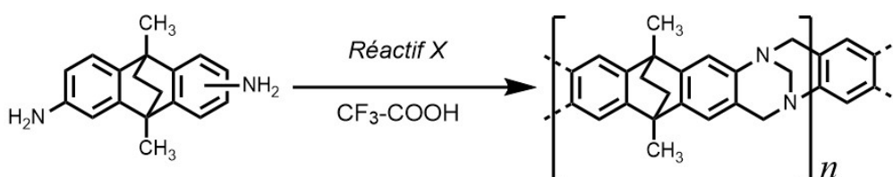
Figure 8 : Synthèse proposée pour le polymère
