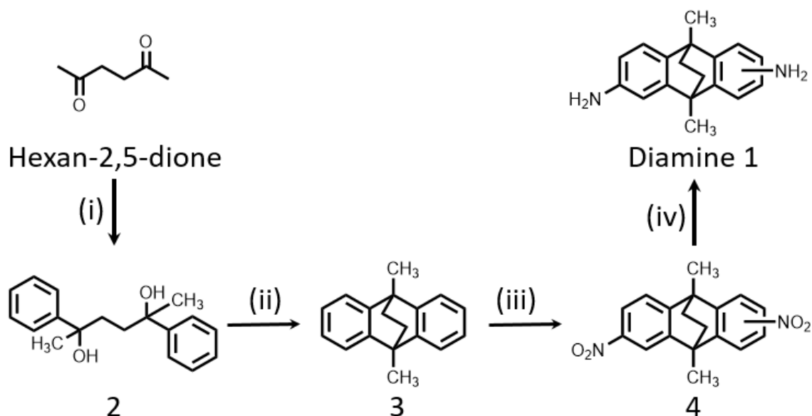
Figure 9 : Synthèse de la Diamine 1. Réactifs, conditions et rendement : (i) \text{PhMgBr} , THF, reflux puis \text{H}_2\text{O(s)} ; (ii) \text{AlCl}_3 , toluène sec, TA puis reflux 48 h, puis \text{H}_2\text{O} , 36 %; (iii) \text{KNO}_3 , anhydride trifluoroéthanoïque, acétonitrile, TA 24 h, 92 %; (iv) \text{N}_2\text{H}_4 \cdot \text{H}_2\text{O} , \text{Ni(Raney)} , diéthyléther reflux, 24 h 100 %.
