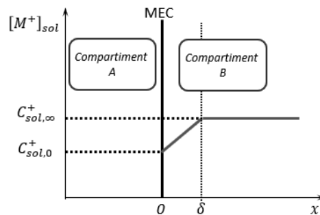
Figure 15 : Profil de concentration en cation M^+ dans l'effluent B au voisinage d'une MEC en régime stationnaire. x : distance à la membrane ; \delta épaisseur de la couche de diffusion. C_{sol,\infty}^+ : concentration en M^+ au-delà de \delta ; C_{sol,0}^+ : concentration en M^+ à la surface de la membrane dans le compartiment B.
