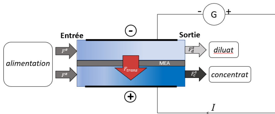
Figure 16 : Représentation schématique d'une unité de concentration de lactate.
