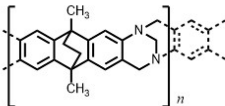
Figure 5 : Formule du polymère à microporosité intrinsèque étudié. Le motif répétitif est représenté entre crochet. Pour améliorer la lisibilité, la connexion à une unité adjacente est représentée en tirets.
