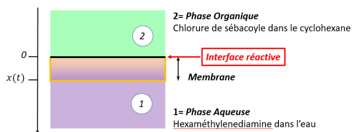
Figure 2 : Coupe transversale schématisée de la membrane en croissance à l'interface entre la phase aqueuse contenant la diamine et la phase organique contenant le dichlorure d'acyle. La membrane est schématisée par le rectangle orange ; les couleurs mauve et verte reflètent les concentrations respectivement en diamine et en chlorure de sébacoyl.
