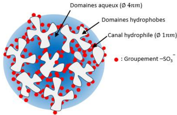
Figure 10 : Représentation schématique du modèle en cluster d'une membrane de Nafion gonflée d'eau. Les groupes hydrophiles sulfonate (en rouge) ne se trouvent que dans les domaines aqueux. \varnothing indique le diamètre.
