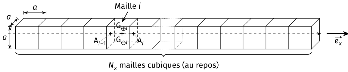
Figure 19 – Échantillon macroscopique de matériau piézoélectrique modélisé par N_x mailles cubiques (au repos) d'arête a .
