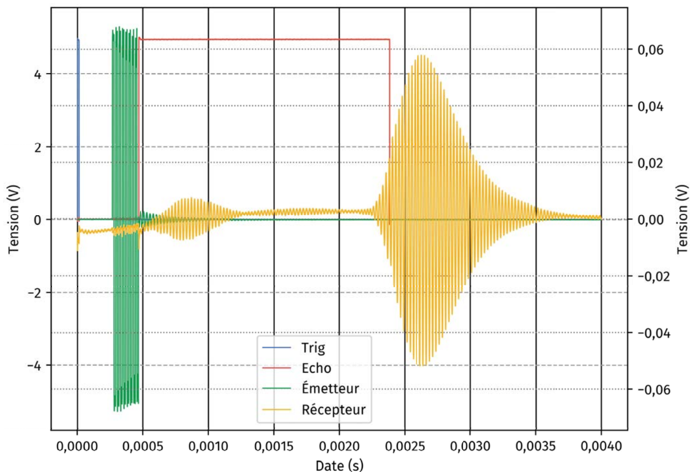
Figure 9 – Évolution temporelle des potentiels des broches « Trig » et « Echo » du module HC-SR04 ainsi que des tensions aux bornes de l'émetteur et du récepteur piézoélectrique. La valeur de la tension aux bornes du récepteur est significativement plus petite que les autres grandeurs mesurées. Afin de pouvoir représenter les quatre grandeurs sur un même graphe, on a utilisé deux échelles différentes pour l'axe des ordonnées : l'échelle de droite se rapporte à la tension aux bornes du récepteur et l'échelle de gauche se rapporte aux trois autres grandeurs.
