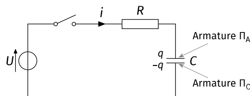
Figure 15 – Schéma du circuit mettant en œuvre le condensateur de capacité C .
