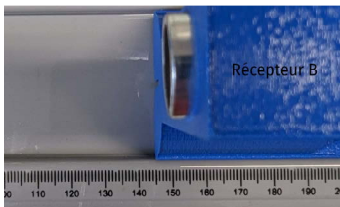
Figure 4 – Le récepteur A est à la graduation 0 mm. L'abscisse du récepteur B est mesurable sur la photo ci-dessus. Les deux tensions visualisées sur les voies 2 et 3 sont en phase.
