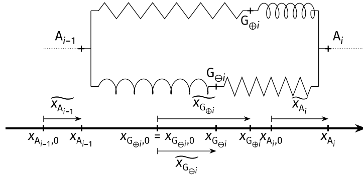
Figure 21 – Déformation de la maille sous l'action d'une contrainte et d'un champ électrique \vec{E} = E\vec{e}_x : écarts aux abscisses de repos.
