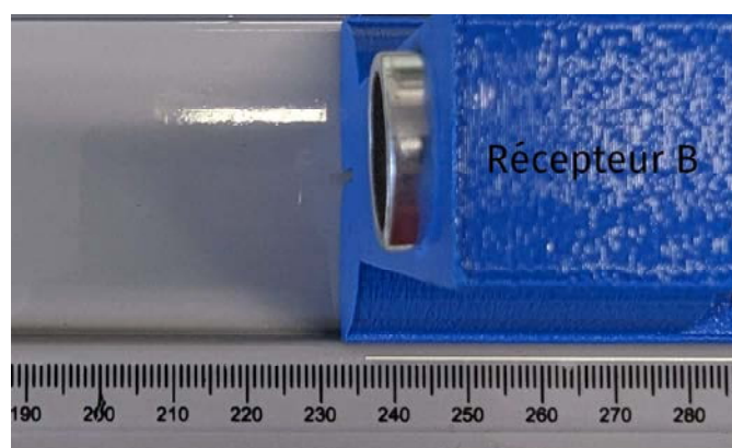
Figure 5 – Le récepteur A est toujours à la graduation 0 mm. Le récepteur B a été déplacé et sa nouvelle abscisse est mesurable sur la photo ci-dessus. Les deux tensions visualisées sur les voies 2 et 3 sont en phase. Entre la position du récepteur B de la figure 4 et celle-ci, il a été observé dix fois successivement que les courbes des voies 2 et 3 étaient en phase.
