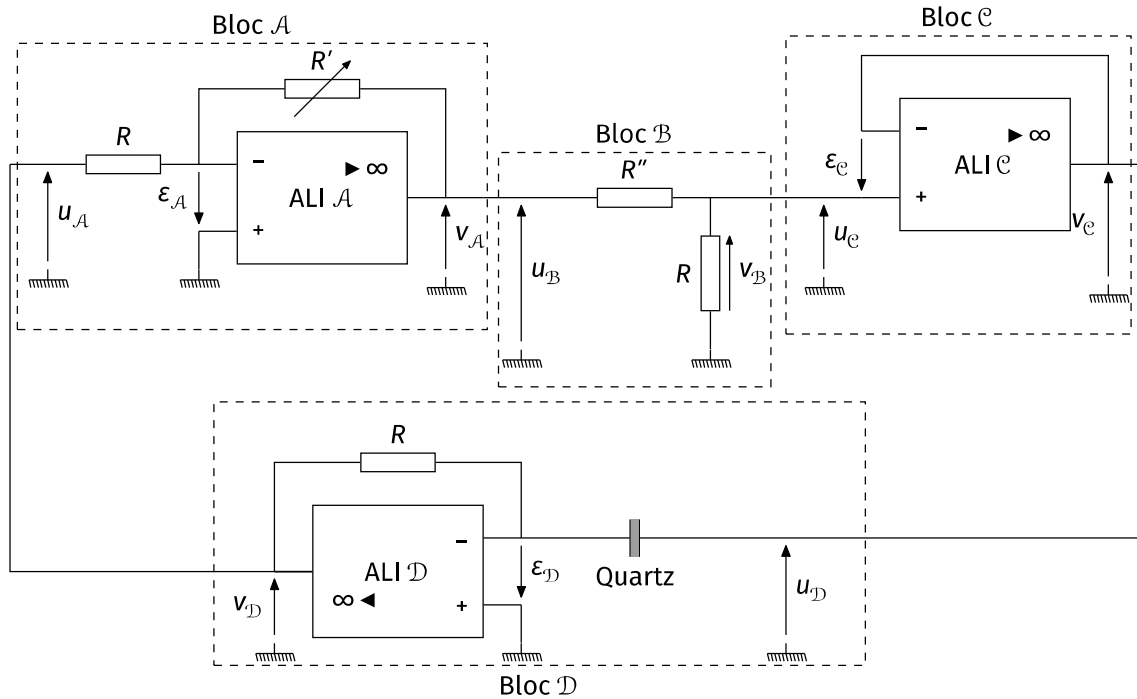
Figure 10 – Schéma d'un oscillateur à quartz.
