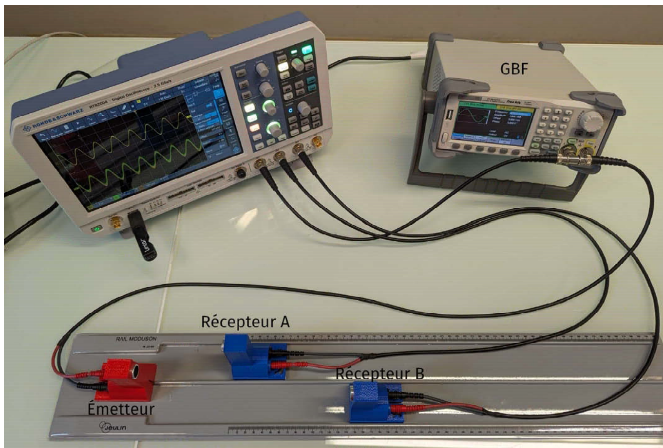
Figure 3 – Montage utilisant un émetteur et deux récepteurs permettant de mesurer la célérité du ultrasons dans l'air.
