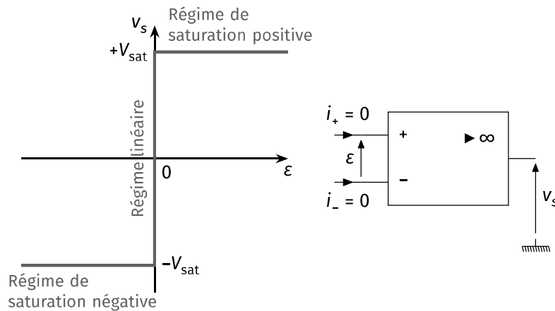
Figure 11 – Caractéristique de transfert d'un ALI idéal fonctionnant dans la limite de gain infini.
