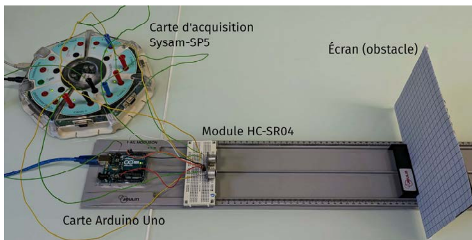
Figure 7 – Montage utilisant un microcontrôleur Arduino et un module HC-SR04 et permettant de mesurer la distance entre le module et un obstacle.
