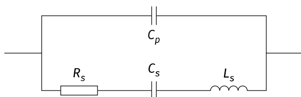
Figure 12 – Dipôle modélisant le comportement électrocinétique d'un quartz.
