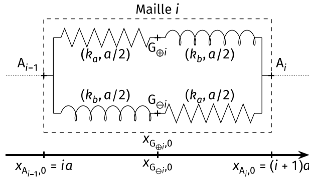
Figure 20 – Modélisation des interactions entre les points G_{\oplus i} , G_{\ominus i} , A_{i-1} et A_i : maille au repos et abscisses au repos. Afin de rendre la figure lisible, les points G_{\oplus i} et G_{\ominus i} ont été décalés verticalement. En réalité, les quatre points G_{\oplus i} , G_{\ominus i} , A_{i-1} et A_i sont alignés horizontalement.
