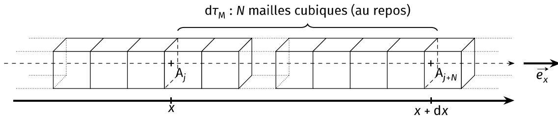
Figure 22 – Volume mésoscopique d\tau_M , compris entre les abscisses x et x + dx , constitué par N mailles cubiques (au repos).
