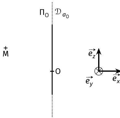
Figure 13 – Schématisation, dans un plan en coupe, de la distribution \mathcal{D}_{\sigma_0} constituée par un plan \Pi_0 uniformément chargé.
