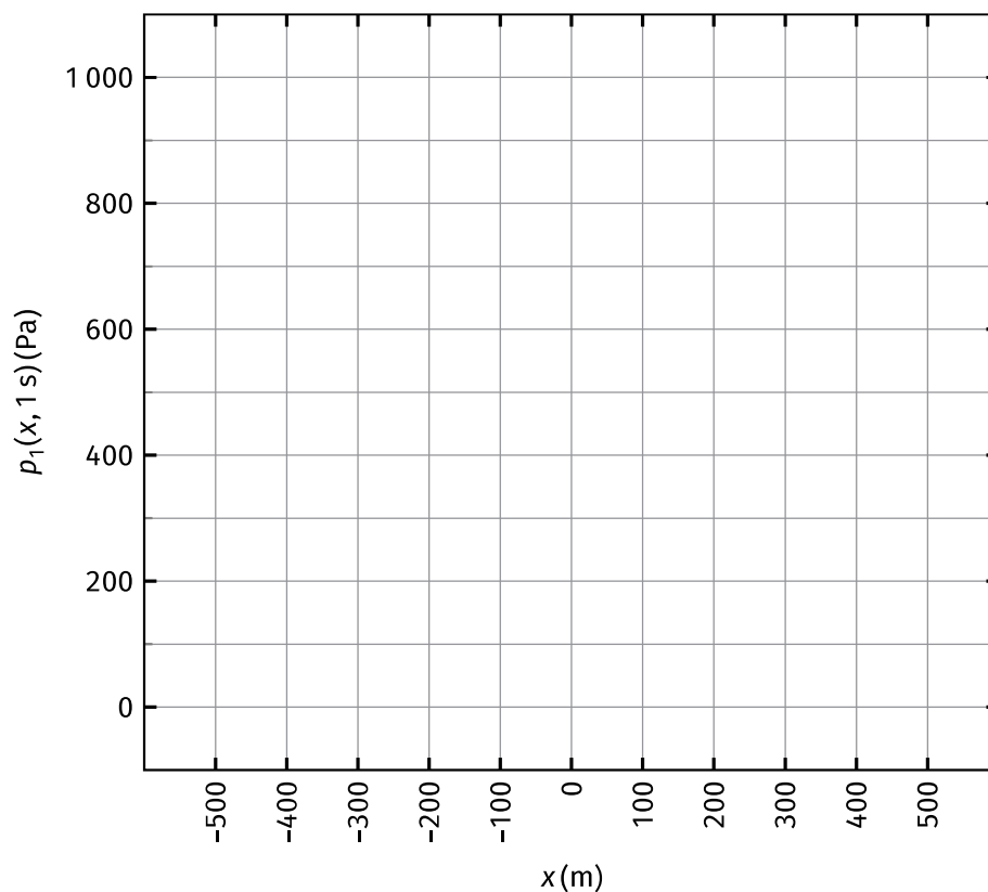
Figure c – Évolution spatiale (à compléter) du champ de surpression p_1(x, t) à la date t = 1 \text{ s} pour le champ de surpression initial représenté dans la figure 2.
