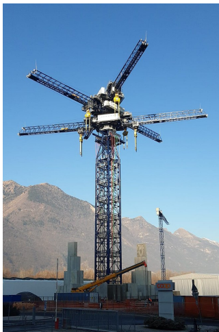
Document 10 : photographie du prototype d'Energy Vault, et schéma de principe qui montre le stockage des blocs de béton.
