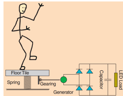
Document 1 : exemple de dispositif de récupération d'énergie des vibrations du sol.
