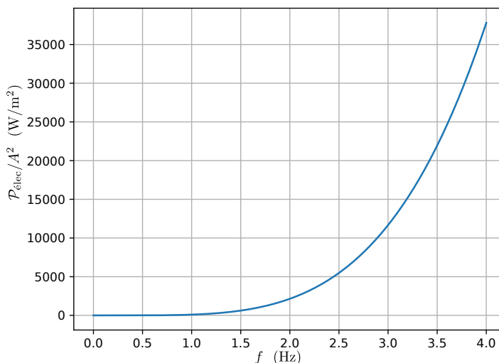
Document 8 : tracé de la puissance électrique moyenne \mathcal{P}_{\text{élec}} produite par le dispositif, divisée par A^2 , d'après le modèle développé dans cet énoncé.
