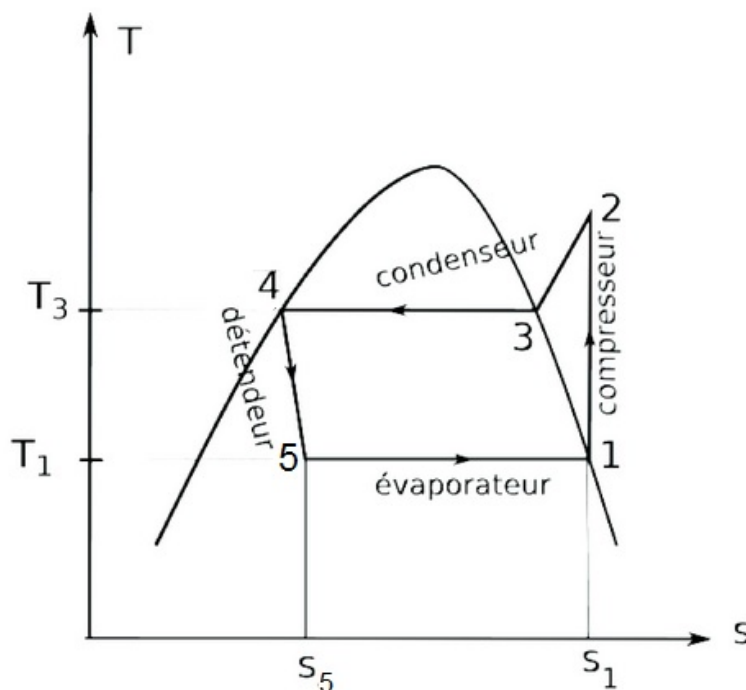
Figure 6 : Allure du diagramme entropique de l'ammoniac. L'entropie massique s est placée en abscisse et la température en ordonnée. On a représenté la courbe d'équilibre liquide-vapeur et placé les différentes étapes du cycle.
