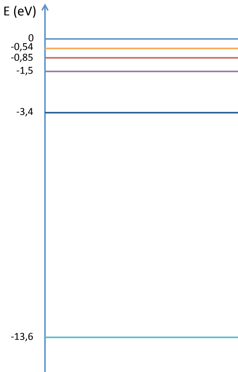
Figure 7 : Diagramme énergétique de l'atome d'hydrogène
