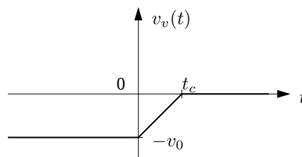
FIGURE 3 – Évolution de la vitesse v_v(t) du véhicule
