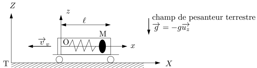
FIGURE 2 – Modélisation du dispositif de détection des chocs installé dans le véhicule
