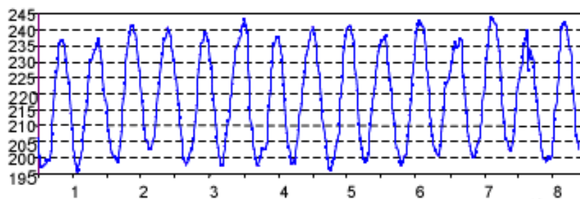
FIGURE 3 – Relevé en laboratoire de l'altitude Z_e(t) (en mm) de la hanche lors de la marche d'un homme à 5 km/h sur un tapis roulant en fonction du temps (en s)
