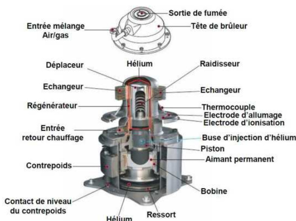
FIGURE 2 – Vue du cogénérateur étudié
